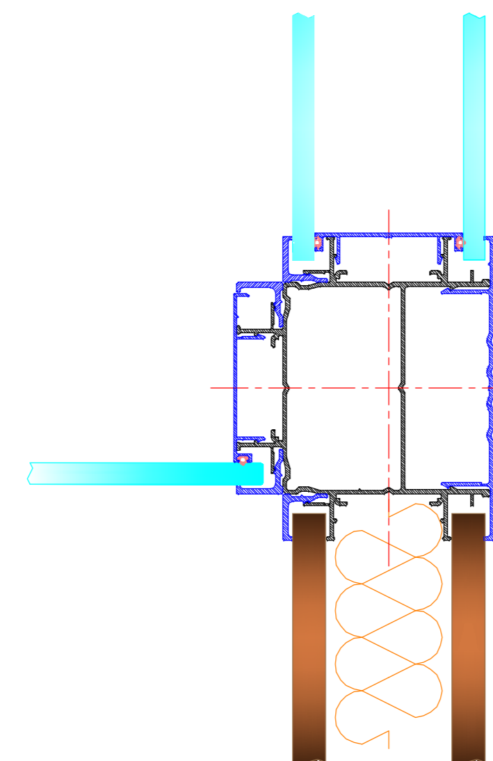
3 départs 3 Ways
